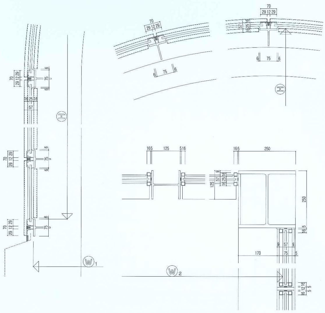
鉛直断面
