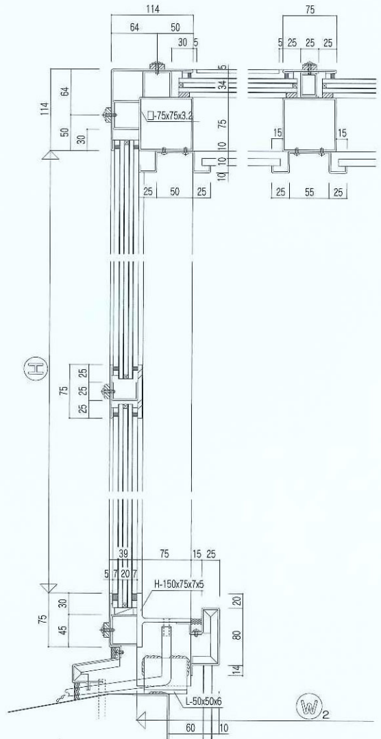
鉛直断面
