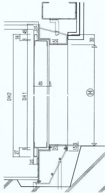
鉛直断面
