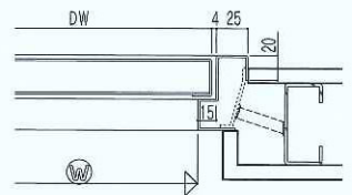
水平断面
