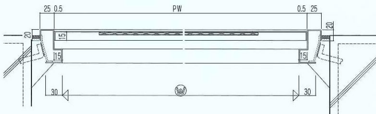
扉部通風口水平断面 (エキスパンドメタル)
