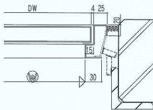
水平断面
