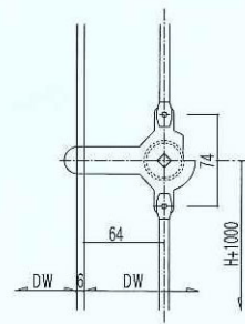
ロックハンドル
