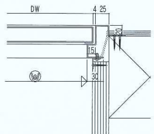
水平断面
