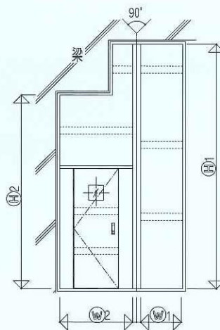
パネル付(コーナー)タイプ
