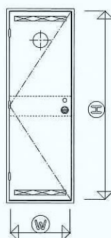
全面片開きタイプ
