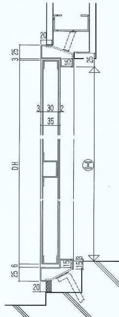
鉛直断面
