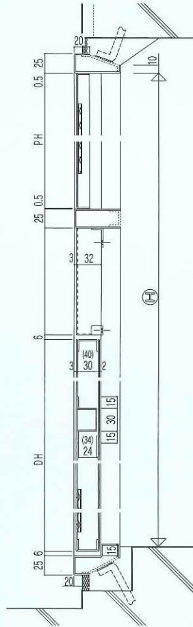
下段片開き鉛直断面
