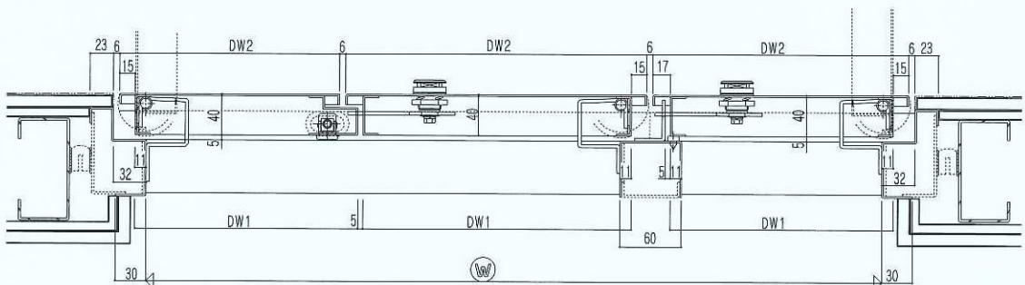
水平断面
