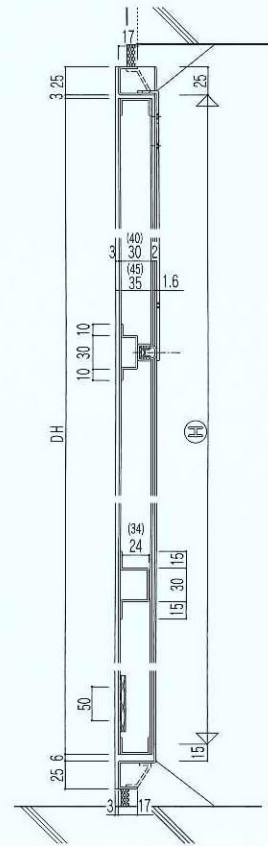
全面片開き鉛直断面
