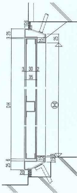
鉛直断面
