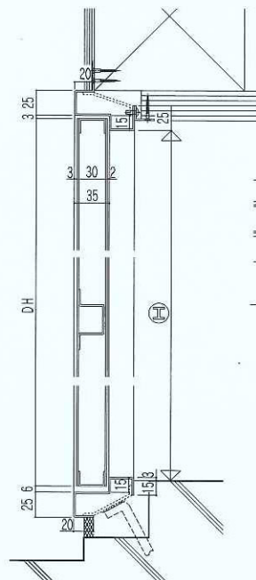
鉛直断面
