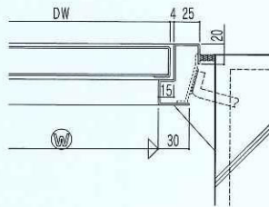
水平断面
